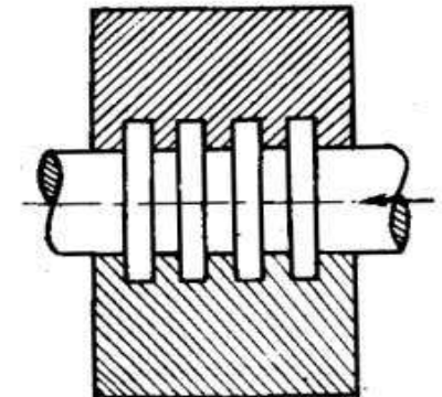
(d) Thrust bearing, multiple collar
